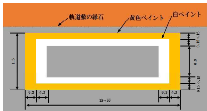
図例(2) 設置例
