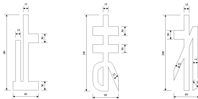
寸法図
